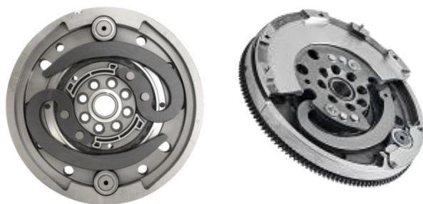
Valeo VBLADE™ DVA
